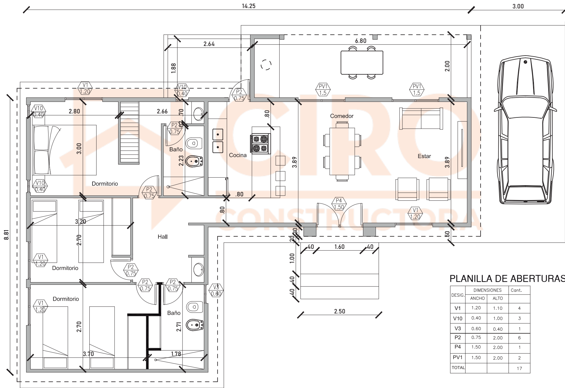
PLANTA ESC 1:75
